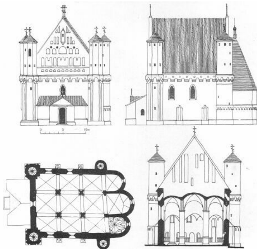
Sinkovičių Šv. Mykolo Arkangelo cerkvės planas
